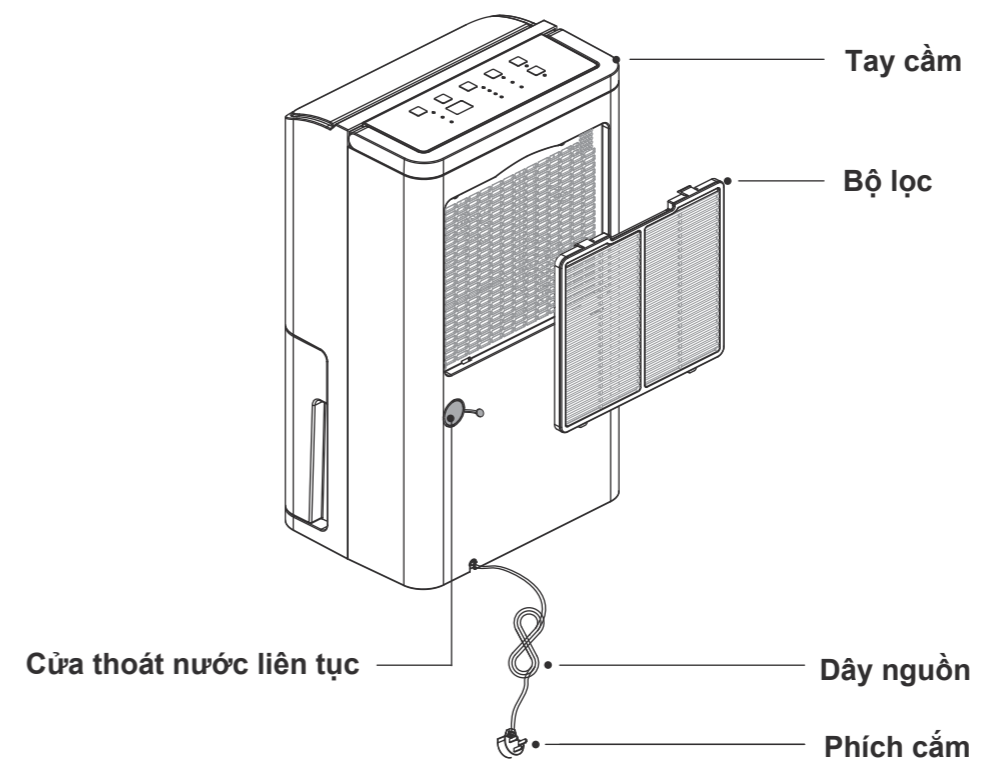
Hình chiếu sau
